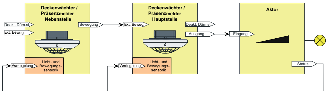
Bild 27: Applikationsbeispiel Haupt- und Nebenstelle ohne Dämmerungsstufenauswertung
