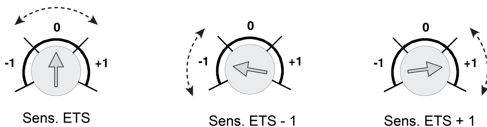
Bild 12: Einstellbereiche des Empfindlichkeitseinstellers am Gerät (-1 <-> 0 <-> +1)
