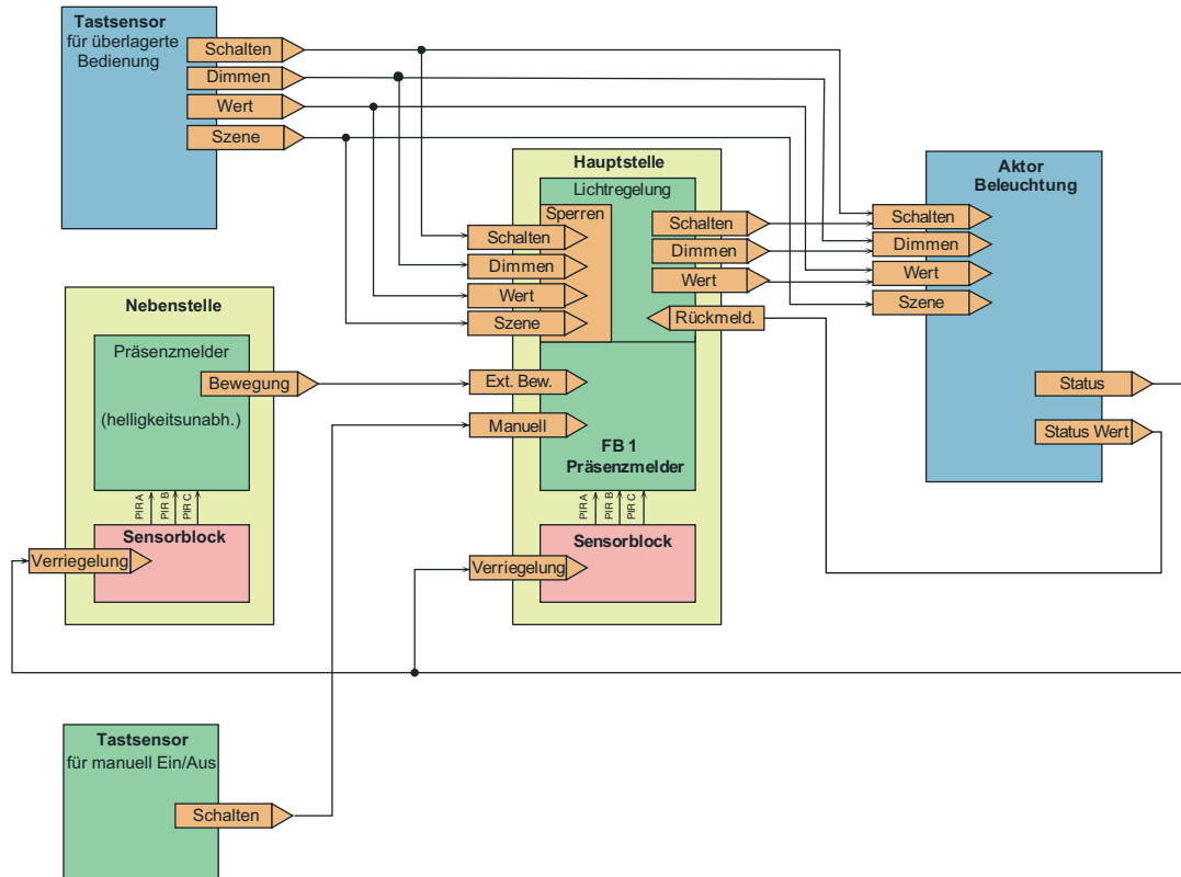
Bild 57: Applikationsbeispiel 1
