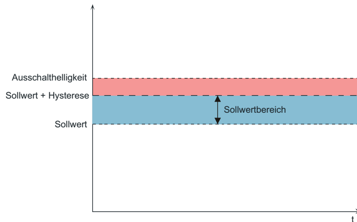
Bild 53: Die Abschalthelligkeit ergibt sich relativ aus dem Sollwert und dem Hysteresewert des Sollwerts
