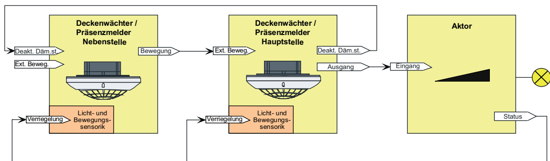
Bild 30: Applikationsbeispiel mit Dämmerungsstufenauswertung in der Hauptstelle und in den Nebenstellen Universal-Lösung für alle Datenformate
