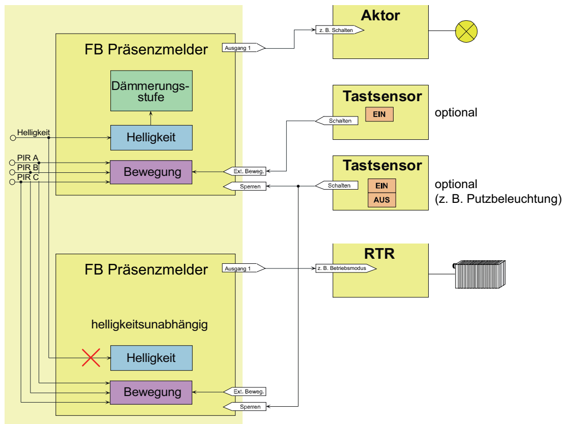
Bild 18: Applikationsbeispiel der Anwendung Präsenzmelder
