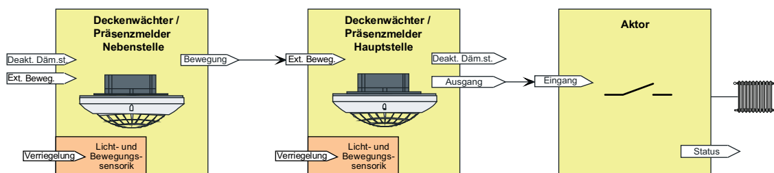
Bild 32: Applikationsbeispiel ohne Dämmerungsstufenauswertung in der Hauptstelle und in den Nebenstellen für Ausgangsfunktionen "Temperaturwertgeber" und "Betriebsmodus Raumtemperaturregler"
