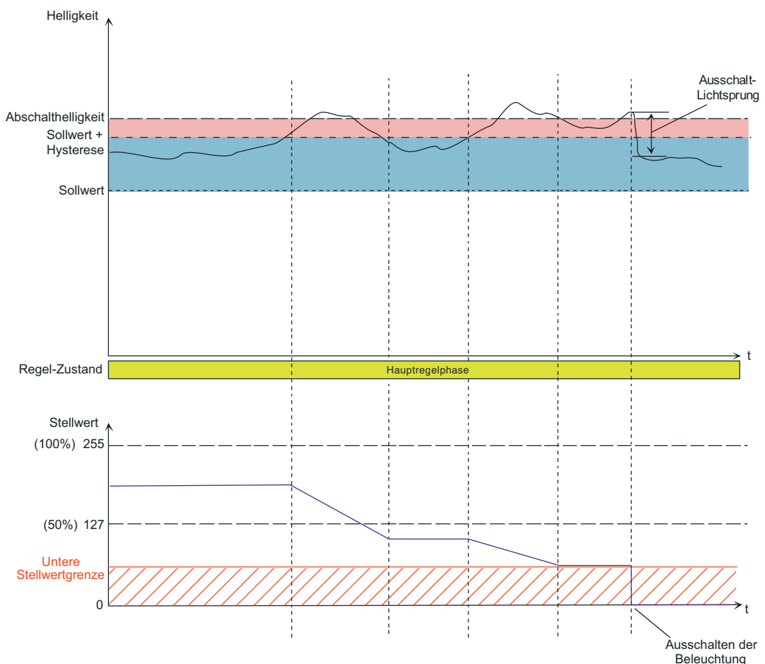
Bild 54: Beispiel einer Stellwertvorgabe bei Auswertung der unteren Stellwertgrenze
