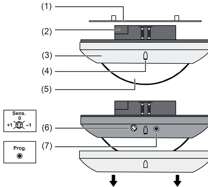
Bild 1: Geräteaufbau
