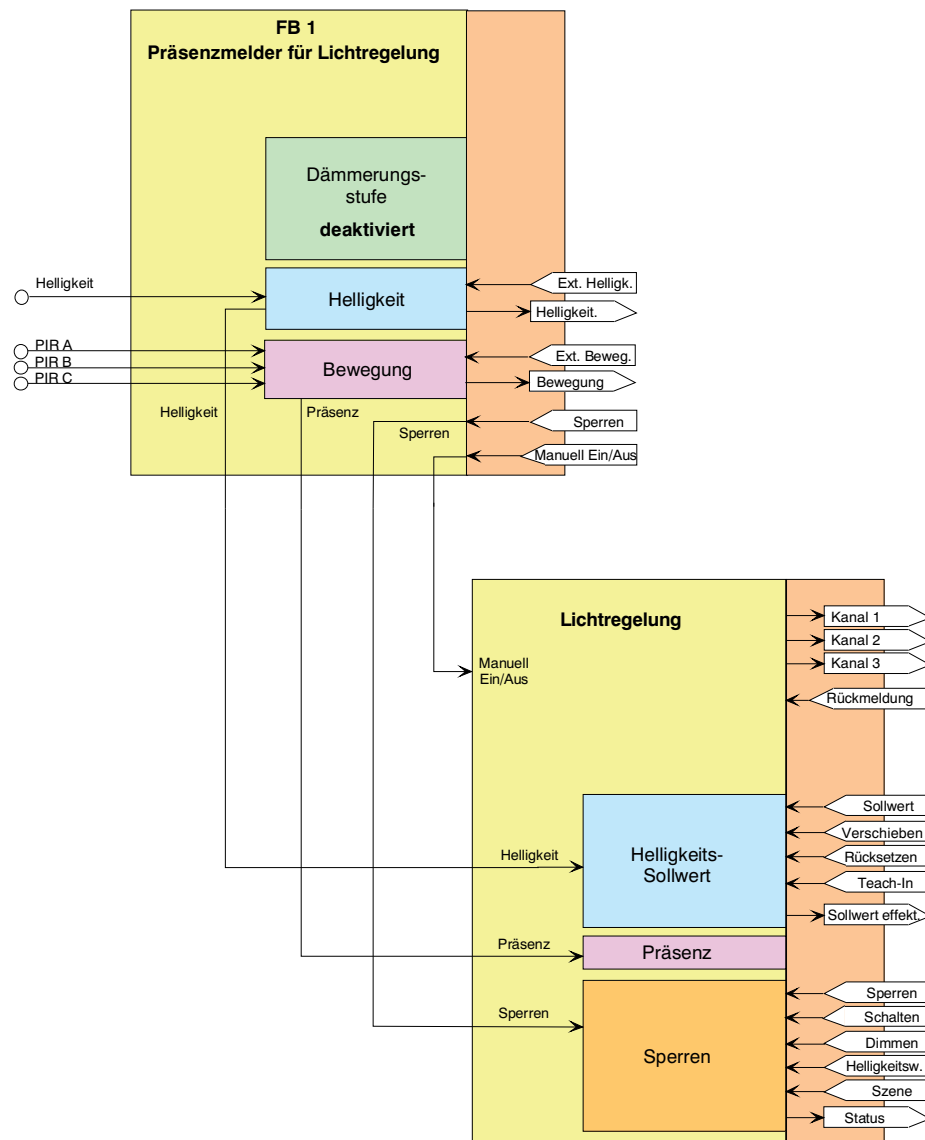
Bild 21: Funktionselemente der Anwendung Präsenzmelder mit Lichtregelung
