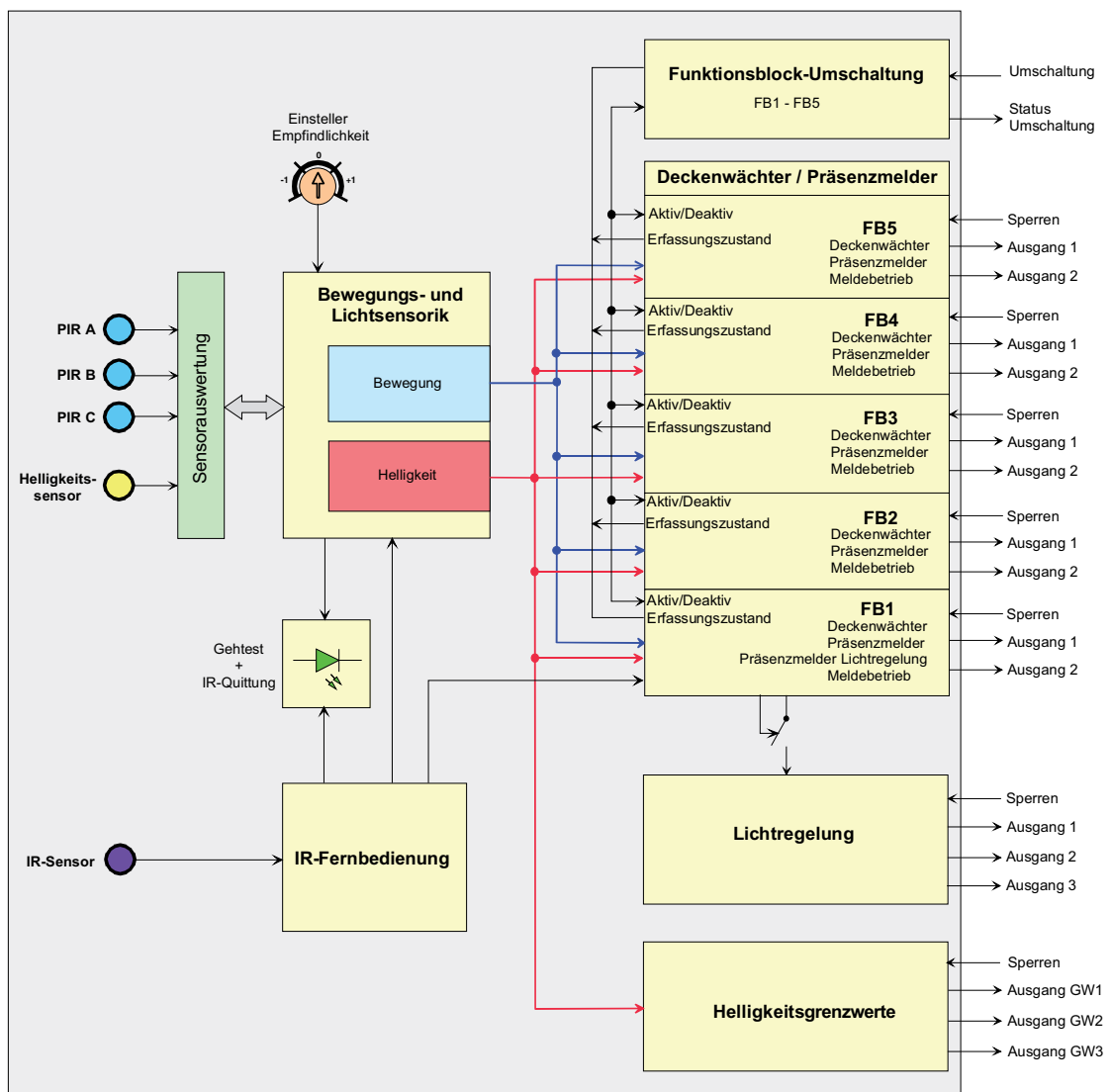
Bild 10: Blockschaltbild aller Funktionen des Geräts
