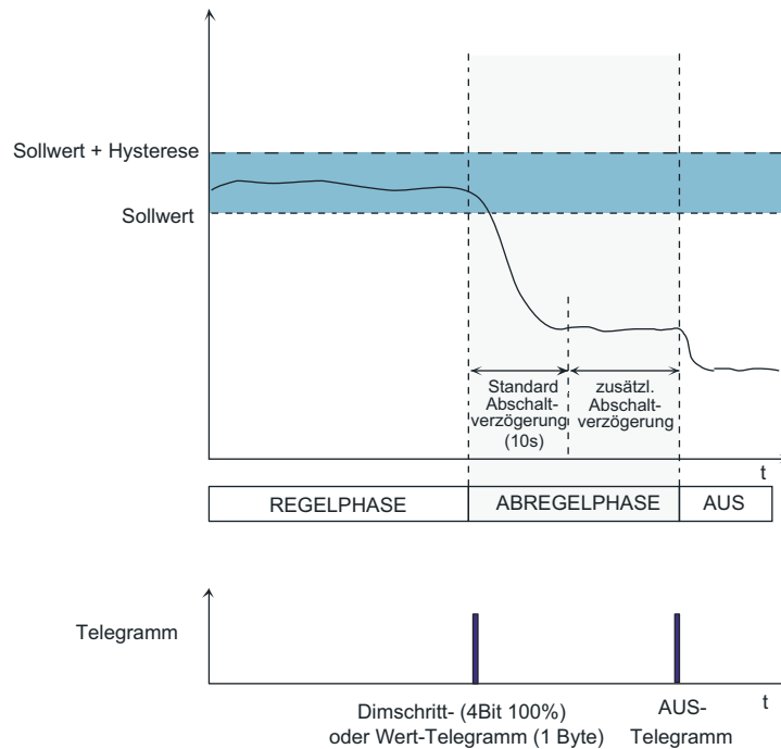
Bild 56: Abregelverhalten mit Wartezeit
