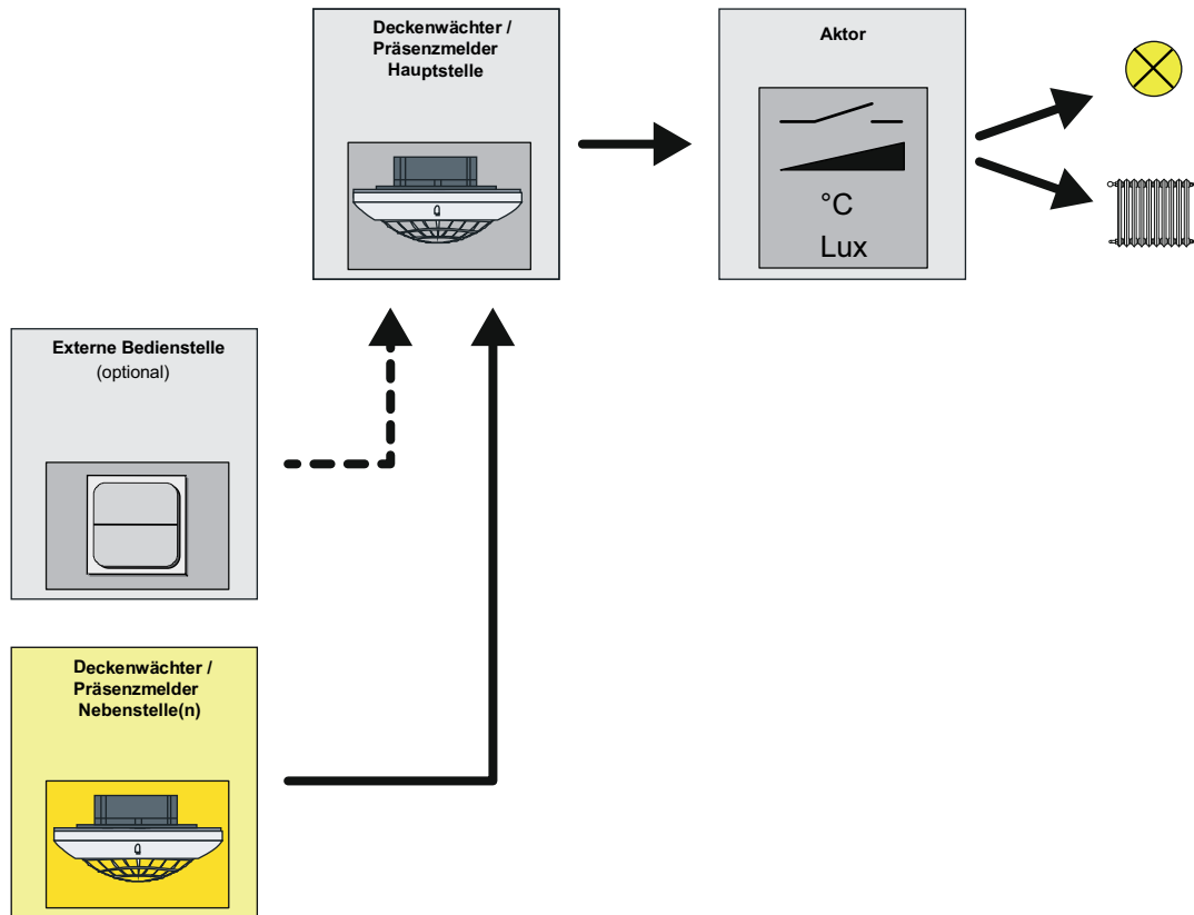
Bild 24: Applikationstyp "Nebenstelle"
