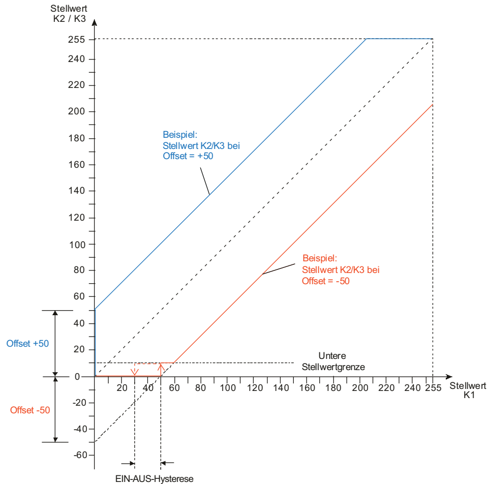
Bild 46: Stellwerte Kanäle 2 oder 3 abhängig vom Stellwert Kanal 1 Verfahren 1: Fester Offset bei zunehmendem Stellwert
