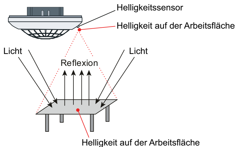
Bild 13: Helligkeitsermittlung durch Messung von reflektiertem Mischlicht aus Kunst- und Tageslichtanteil
