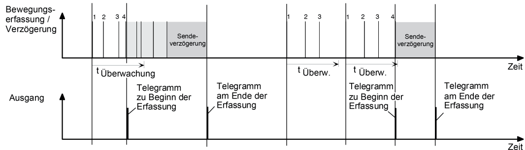
Bild 20: Bewegungsauswertung beim Melder
