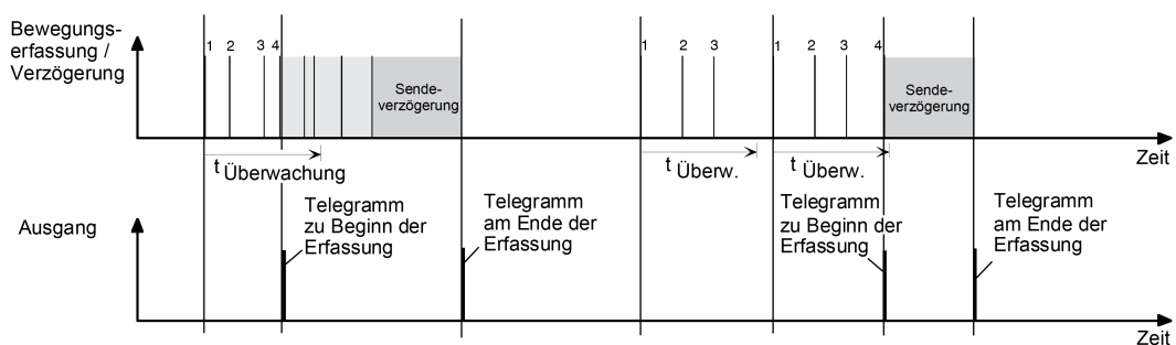
Bild 38: Bewegungsauswertung beim Melder
