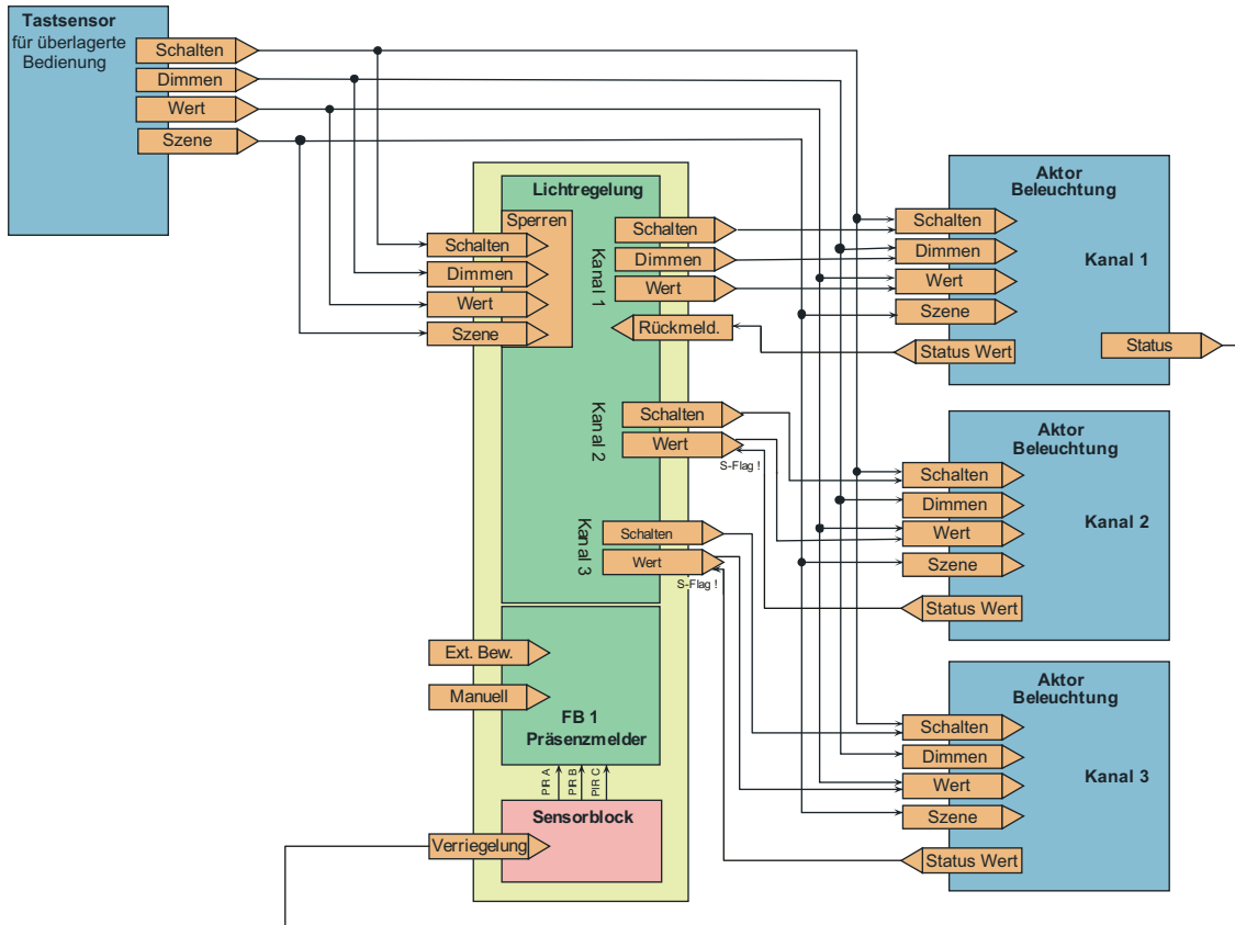
Bild 58: Applikationsbeispiel 2 Funktionsblock 1 als Präsenzmelder für interne Lichtregelung mit 3 Beleuchtungskanälen und Tastsensor für überlagerte Bedienung
