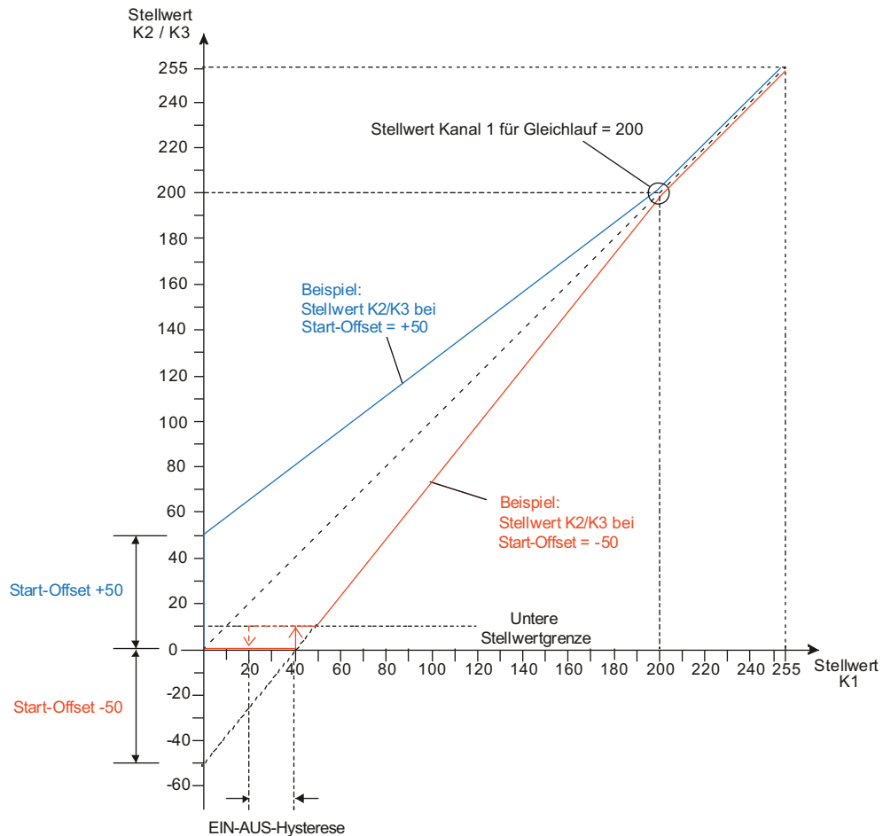
Bild 48: Stellwerte Kanäle 2 oder 3 abhängig vom Stellwert Kanal 1 Verfahren 3: Offset abnehmend bei zunehmendem Stellwert
