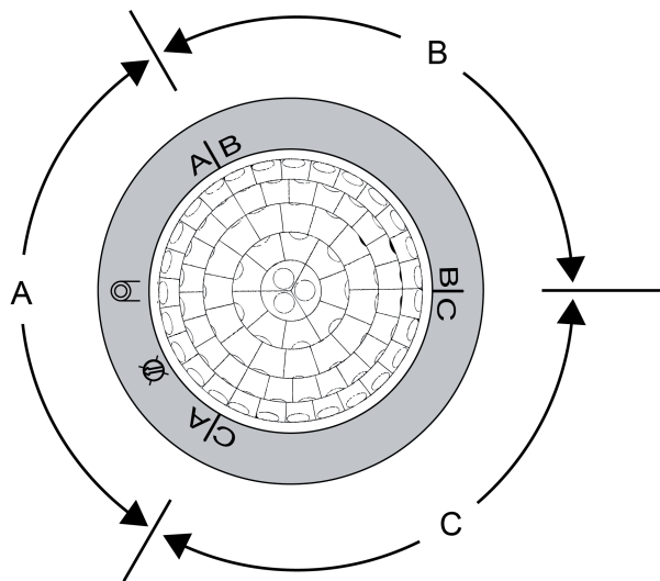
Bild 11: Anordnung der PIR-Sektoren A, B und C
