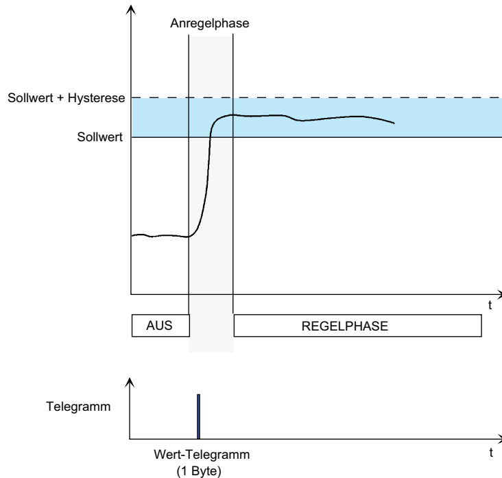
Bild 52: Anregelverhalten mit adaptiver Stellwertvorgabe (1 Byte)
