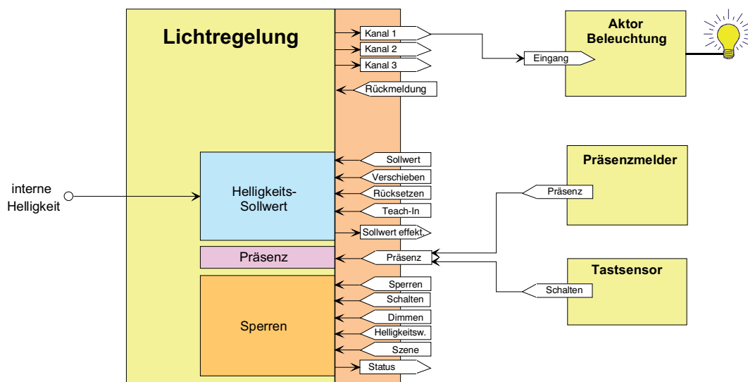
Bild 41: Applikationsbeispiel zur Lichtregelung im autarken Betrieb
