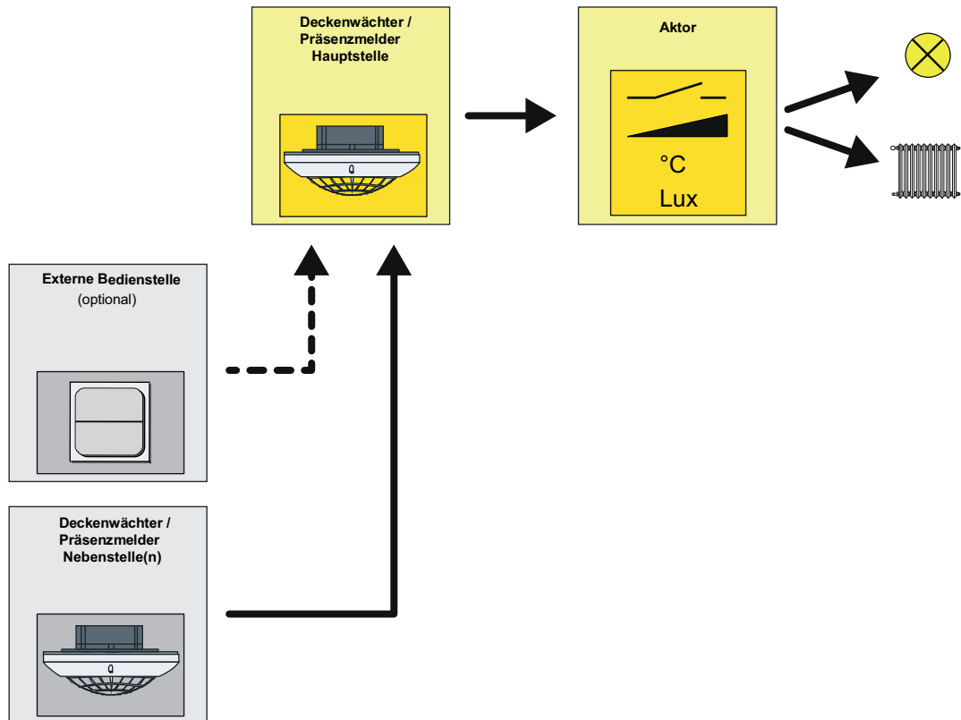
Bild 23: Applikationstyp "Hauptstelle"
