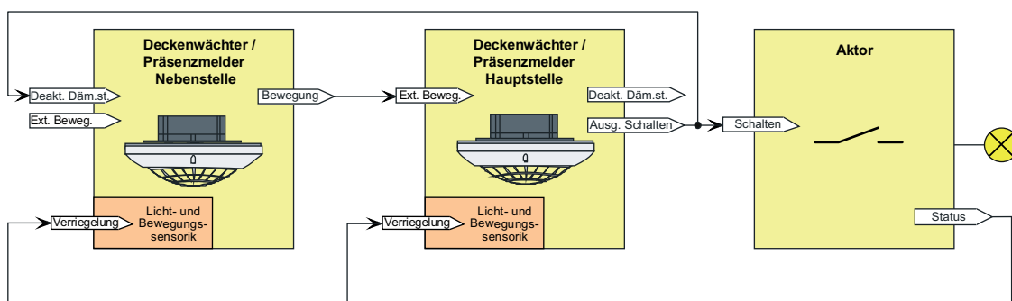
Bild 29: Applikationsbeispiel mit Dämmerungsstufenauswertung in der Hauptstelle und in den Nebenstellen für das Datenformat "Schalten"
