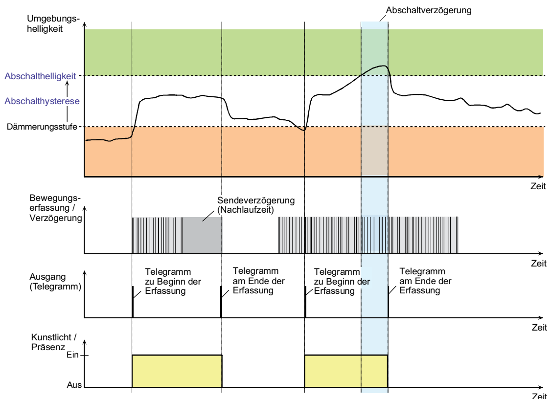
Bild 19: Helligkeits- und Bewegungsauswertung beim Präsenzmelder
