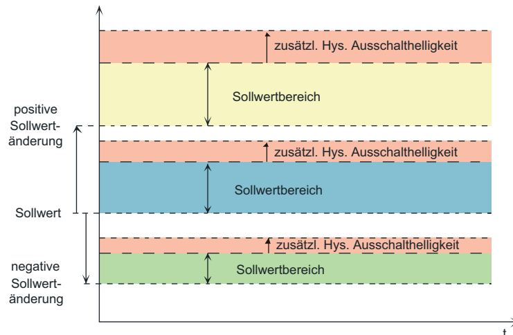
Bild 55: Abhängigkeit der zusätzlichen Hysterese für die Ausschaltelligkeit bei einer Sollwertverschiebung
