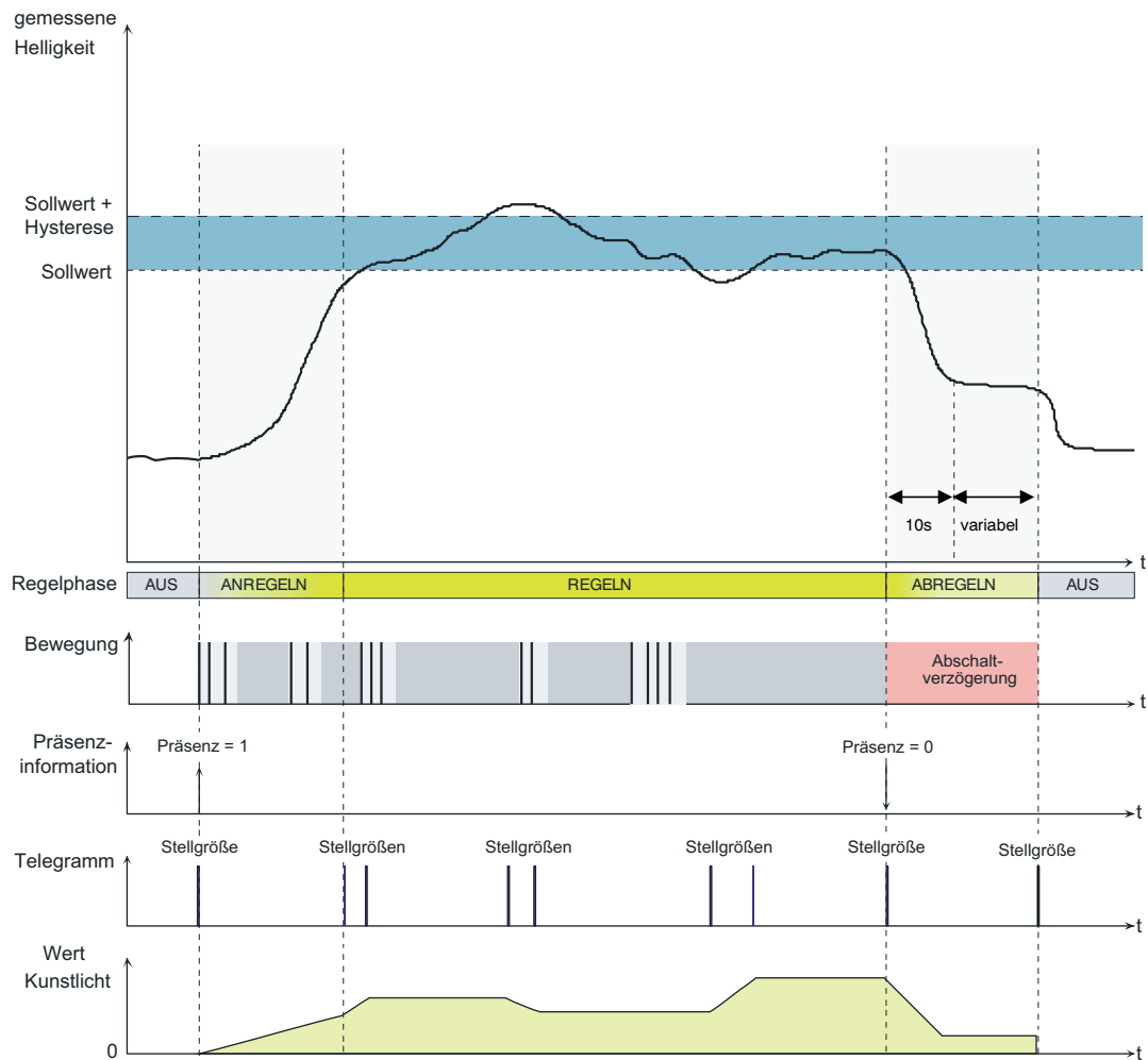
Bild 40: Beispiel eines Regelprozesses mit allen Regelphasen
