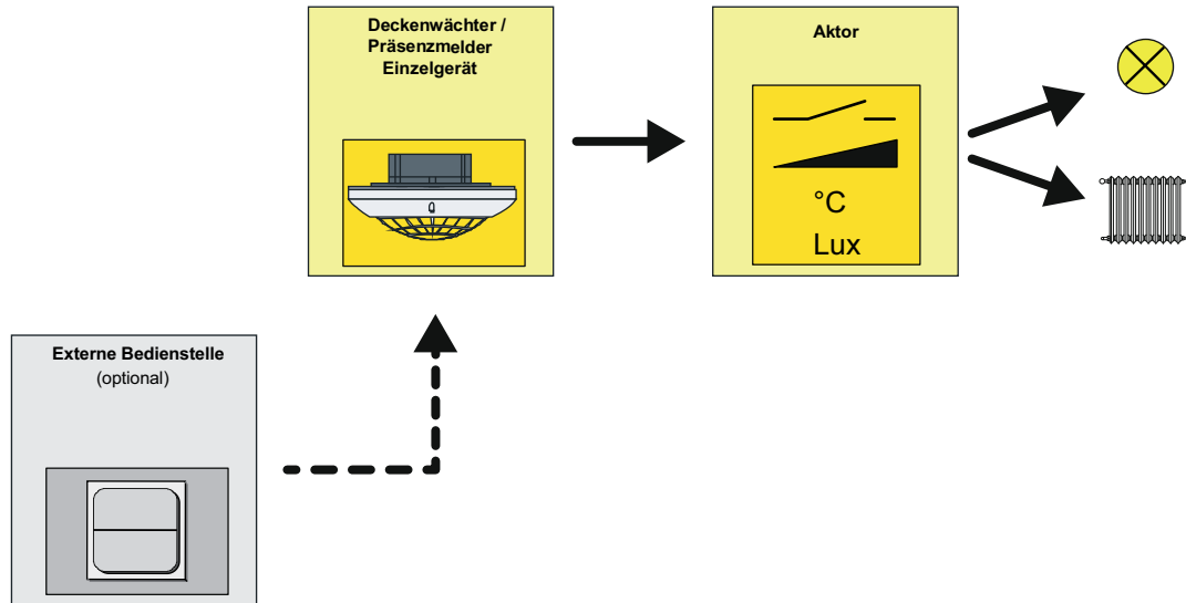
Bild 22: Applikationstyp "Einzelgerät"
