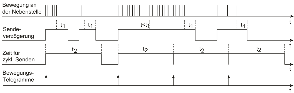
Bild 25: Bewegungssignale einer Nebenstelle
