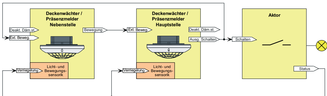
Bild 31: Applikationsbeispiel mit Dämmerungsstufenauswertung in der Hauptstelle und in den Nebenstellen für Ausgangsfunktion "Treppenhausfunktion"
