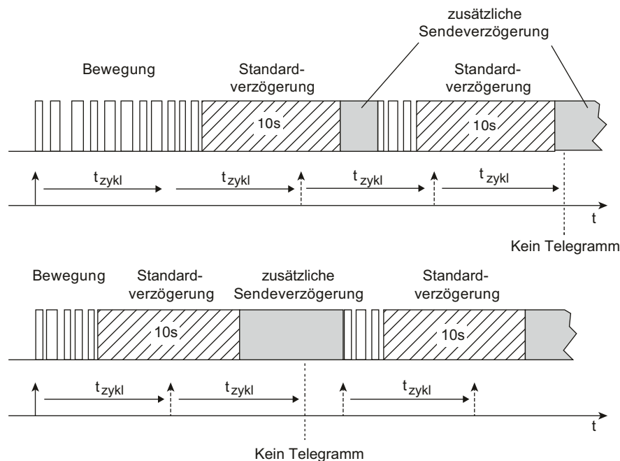
Bild 34: Zyklisches Senden während einer Bewegungserfassung
