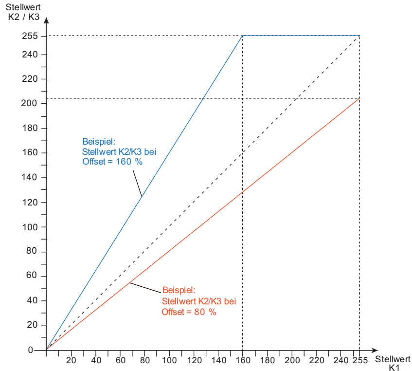
Bild 47: Stellwerte Kanäle 2 oder 3 abhängig vom Stellwert Kanal 1 Verfahren 2: Offset zunehmend bei zunehmendem Stellwert
