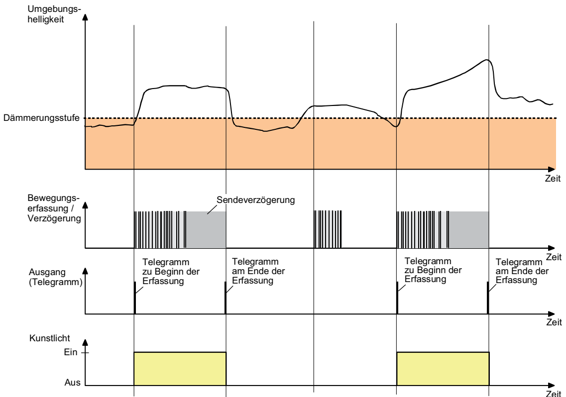
Bild 17: Helligkeits- und Bewegungsauswertung beim Deckenwächter
