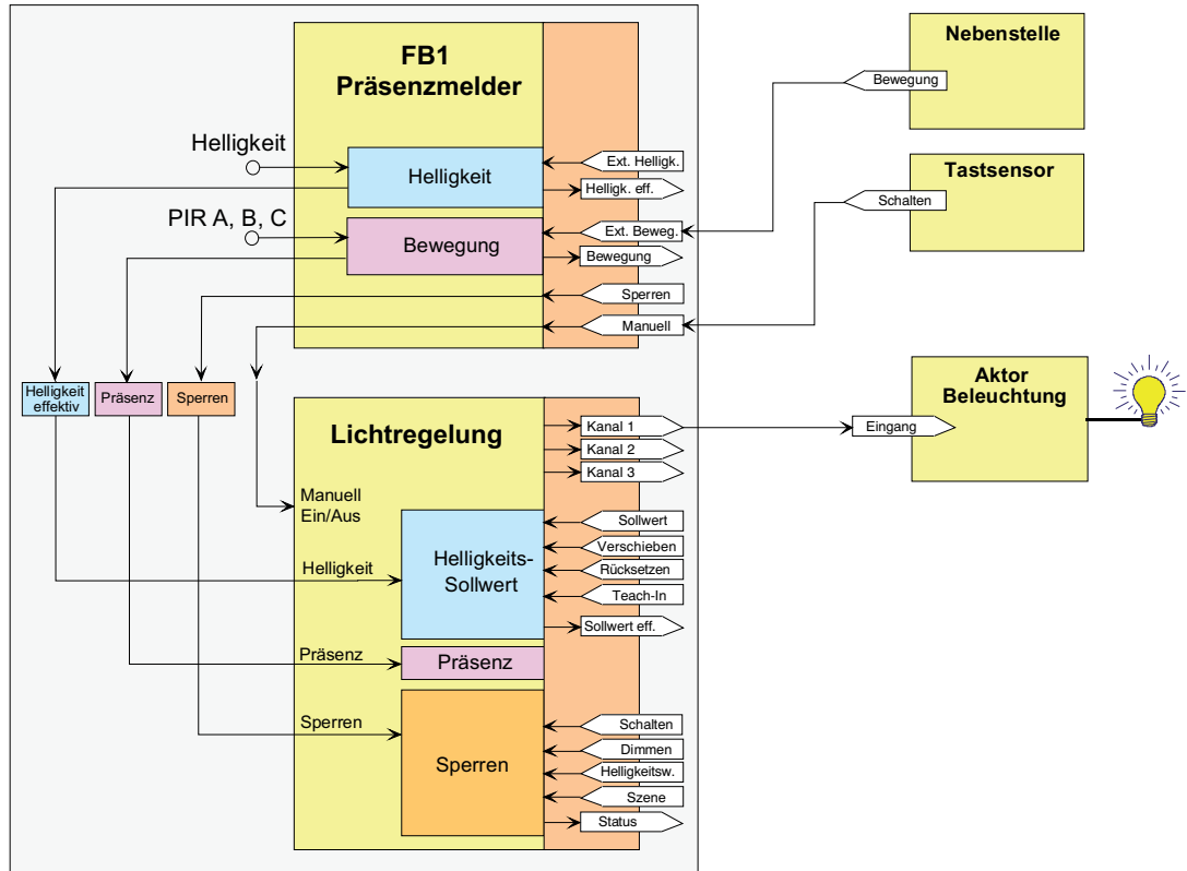
Bild 42: Applikationsbeispiel zur Lichtregelung in Kombination mit dem Funktionsblock 1
