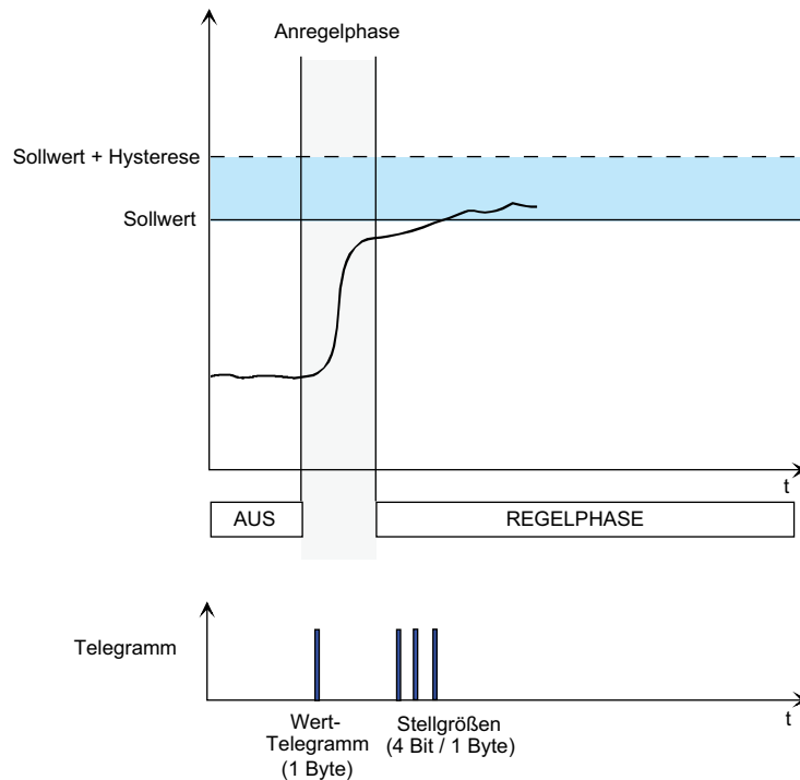
Bild 51: Anregelverhalten mit absoluten Wert-Telegrammen (1 Byte)
