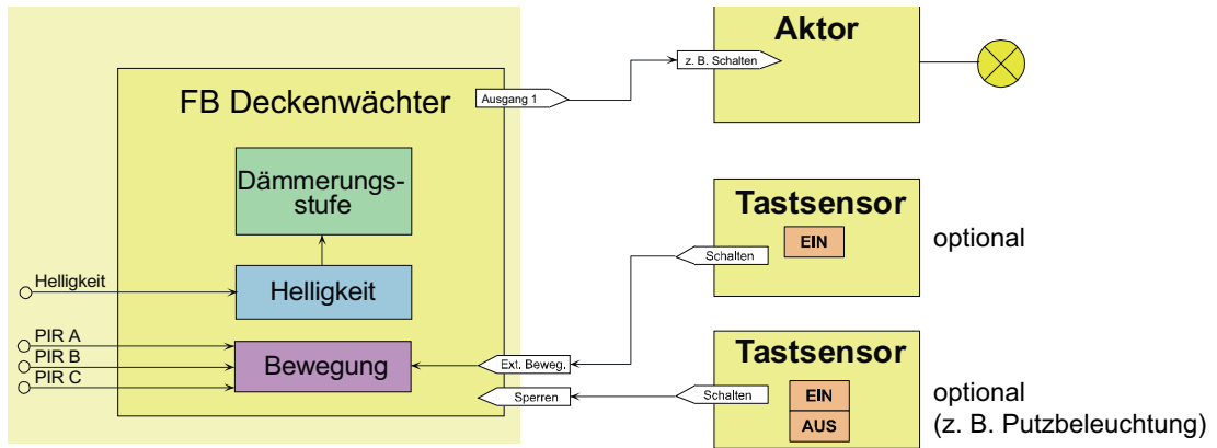
Bild 16: Applikationsbeispiel der Anwendung Deckenwächter
