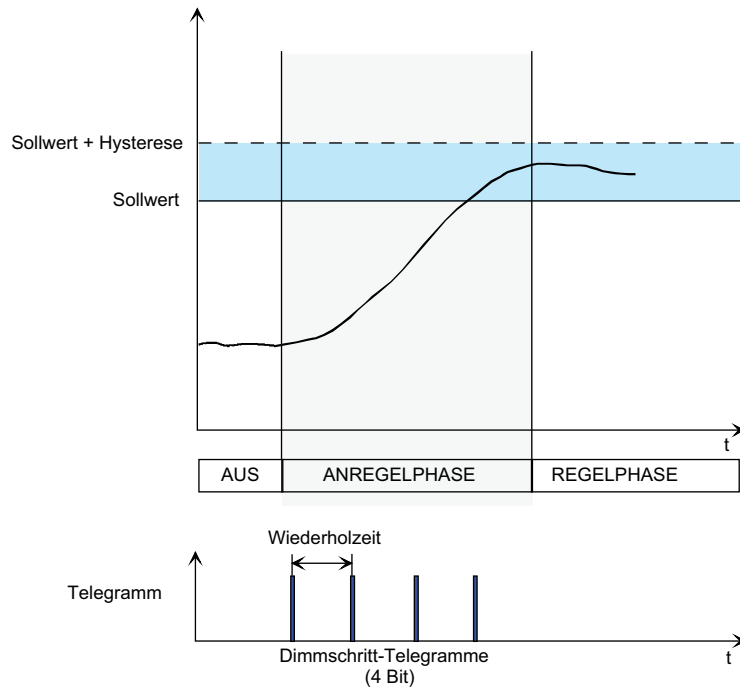
Bild 50: Anregelverhalten mit relativen Dimmschritt-Telegrammen (4 Bit)
