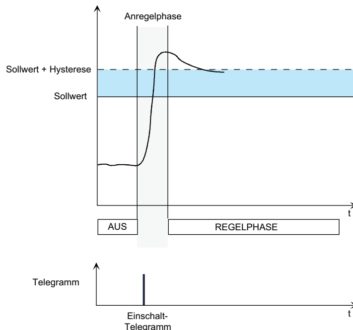
Bild 49: Anregelverhalten mit Schalt-Telegramm (1 Bit)
