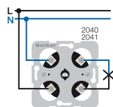
Bild 1: Ausschaltung 2-polig
