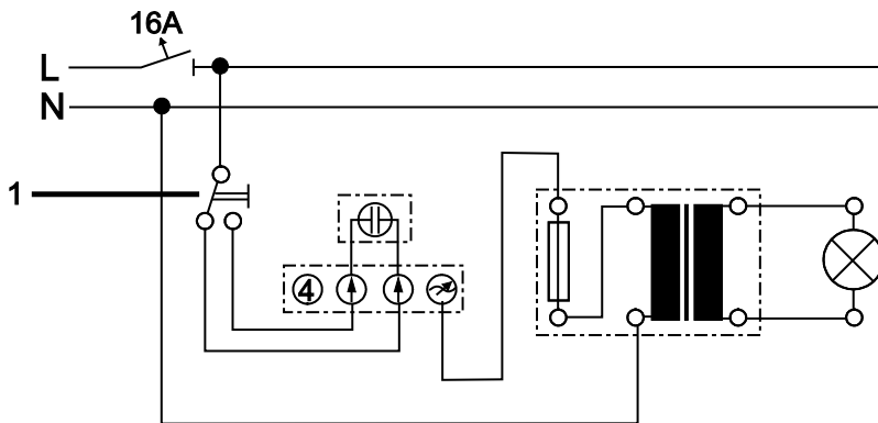
Abb. 2: Schaltbild
