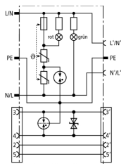
Principalschaltbild DPRO 230 NT
