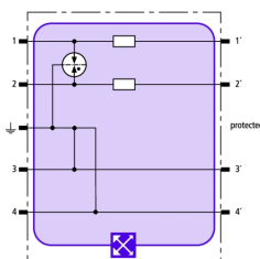
Prinzip Schaltbild BXT ML2 B 180
