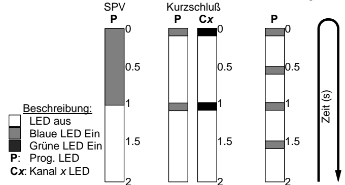
Abb 2. Fehlercodes-LED
