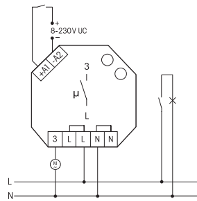
Ventilatorsteuerung über Kleinspannungs-Türkontakt, Licht getrennt geschaltet
