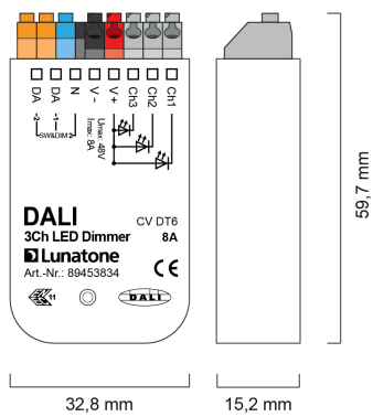
Geometrie Dose
