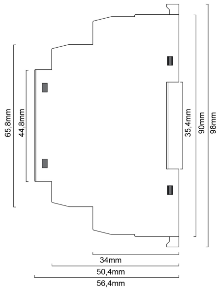
Geometrie Hutschie
