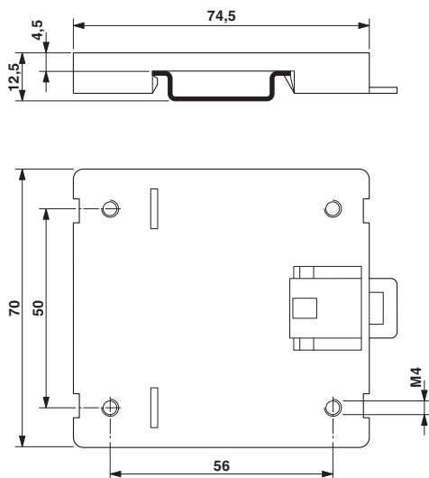
Maßzeichnung
