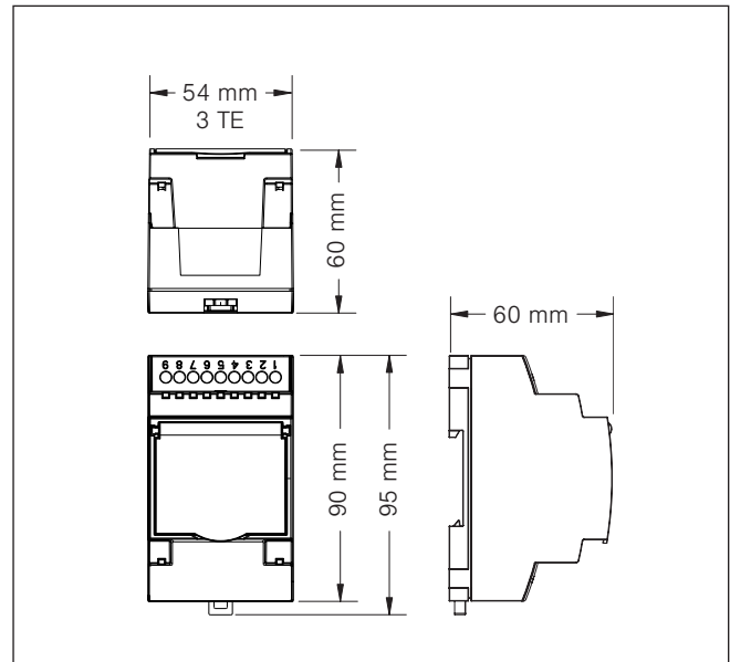
Abb. 6 Abmessungen Reiheneinbaugeschäfte 3 TE für KNX SA 16M230 SMI REG und KNX SA 16MDC SMI LoVo REG.
