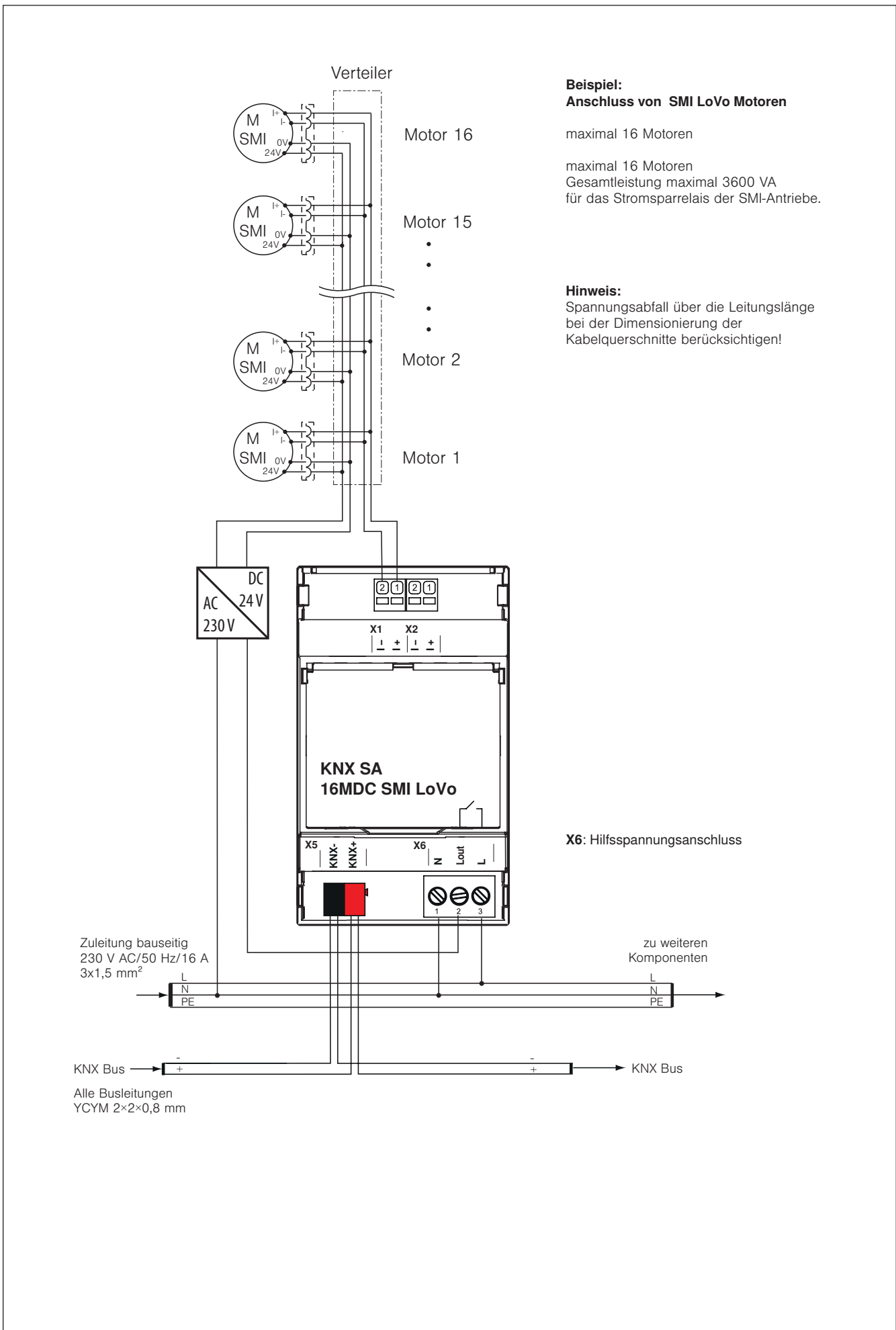
Abb. 8 Anschlussbeispiel KNX SA 16MDC SMI LoVo REG
