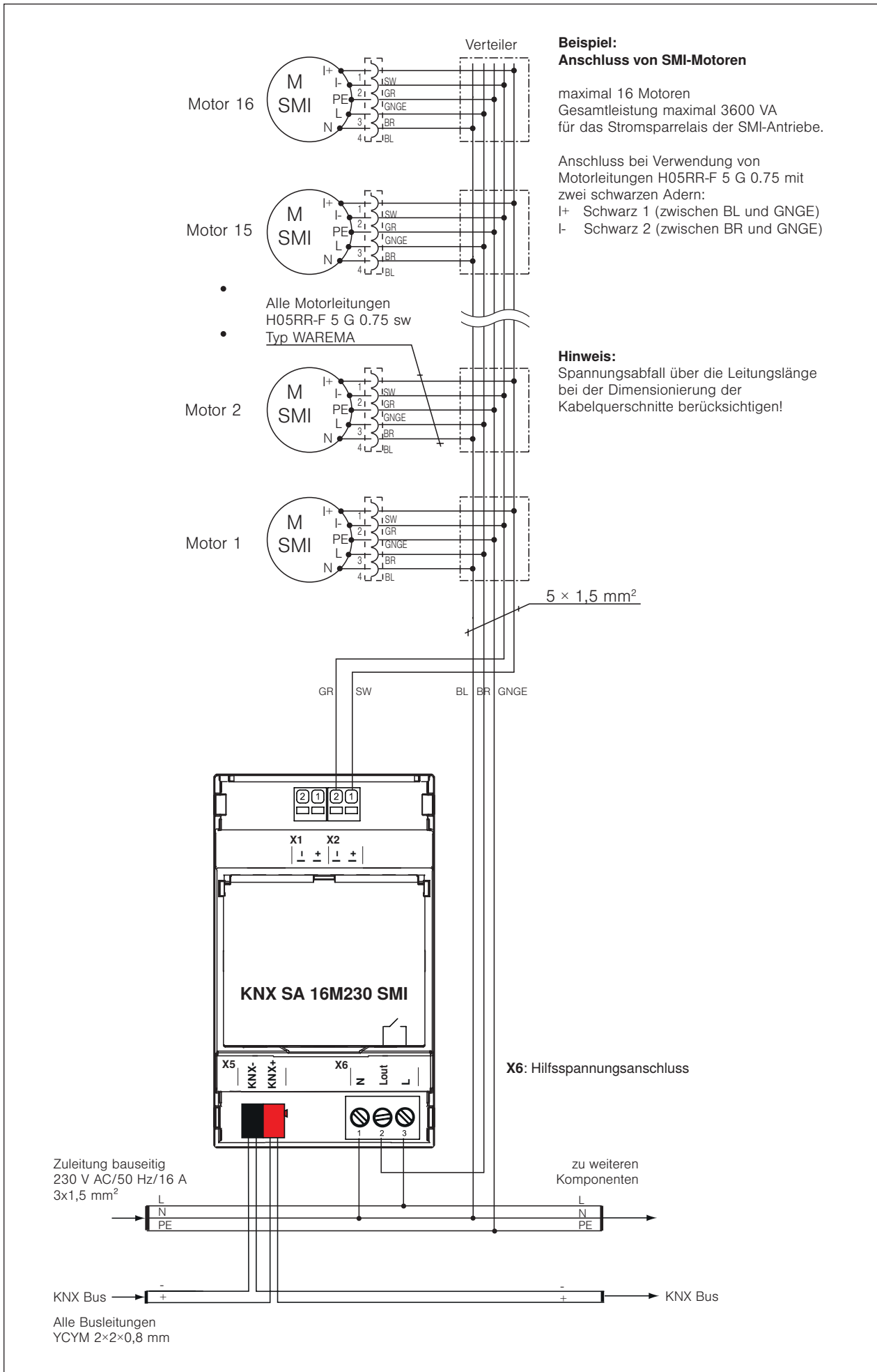
Abb. 7 Anschlussbeispiel KNX SA 16M230 SMI REG
