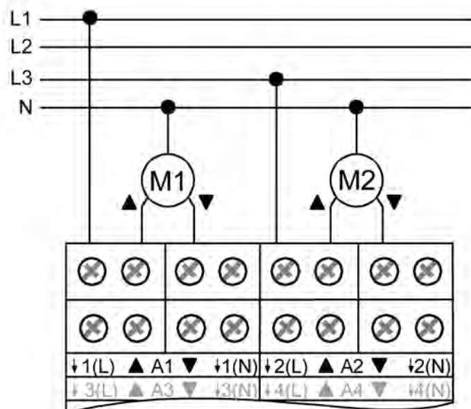
Bild 3: Elektrischer Anschluss für 230 V-Antriebsmotoren
