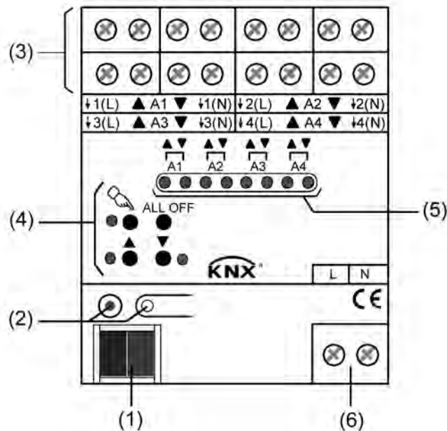
Bild 1: Geräteaufbau
