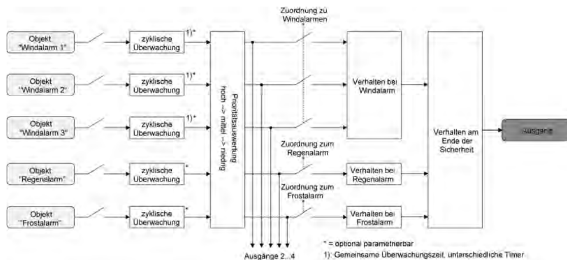
Bild 10: Funktionsschaltbild der kanalorientierten Sicherheitsfunktionen
