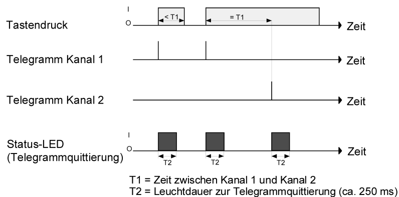
Bild 16: Beispiel zum Bedienkonzept "Kanal 1 oder Kanal 2"
