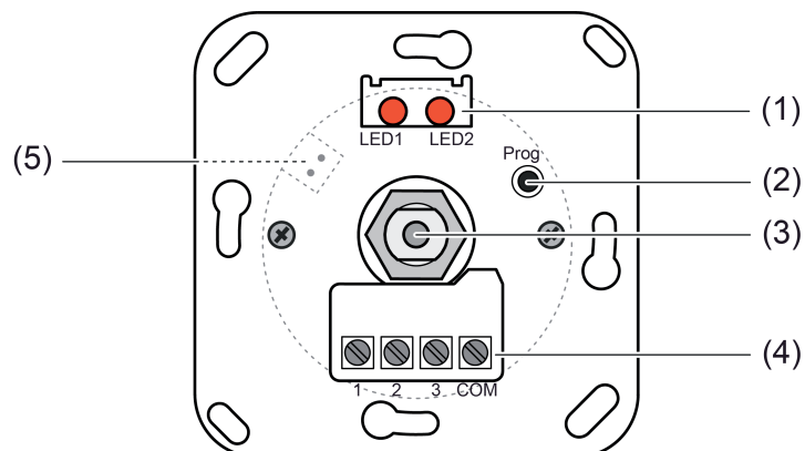
Bild 1: Geräteaufbau (Ansicht Vorderseite)
