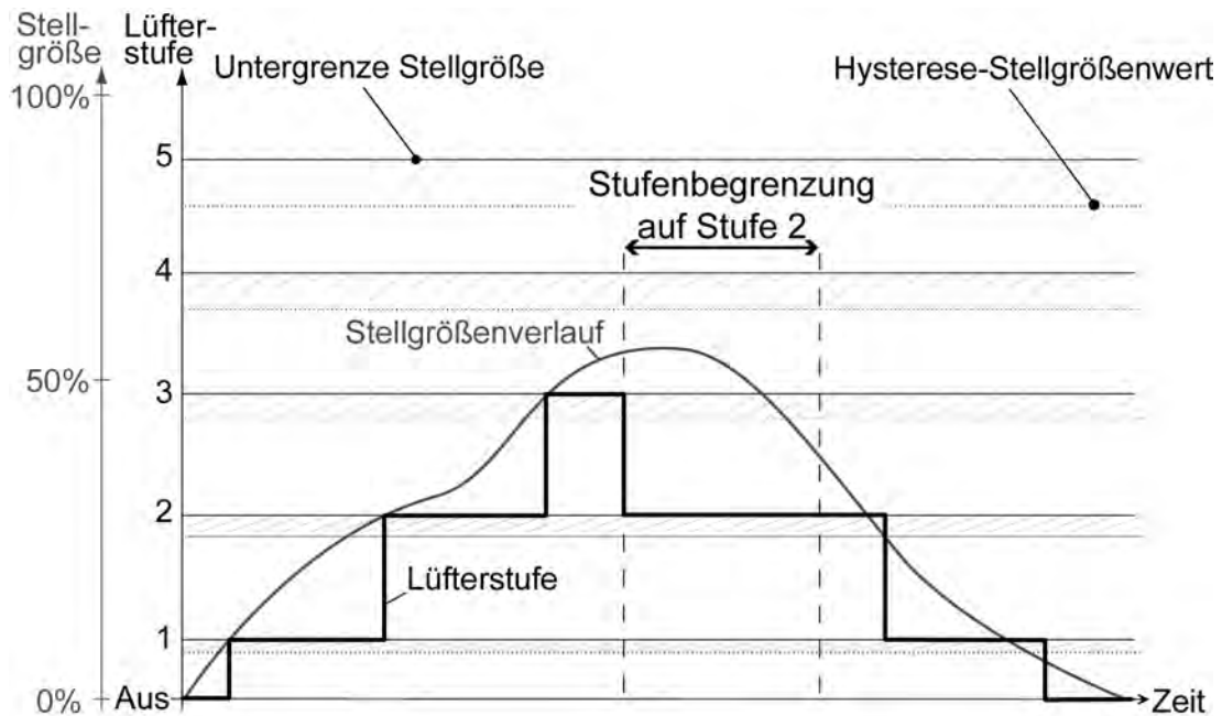
Bild 27: Vereinfachtes Stellgrößenendiagramm zur Verdeutlichung der Reaktion auf eine Lüfterstufenbegrenzung
