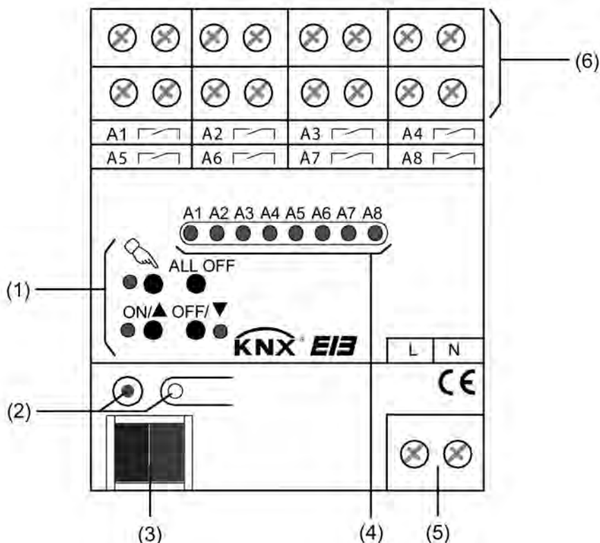
Bild 1: Geräteaufbau
