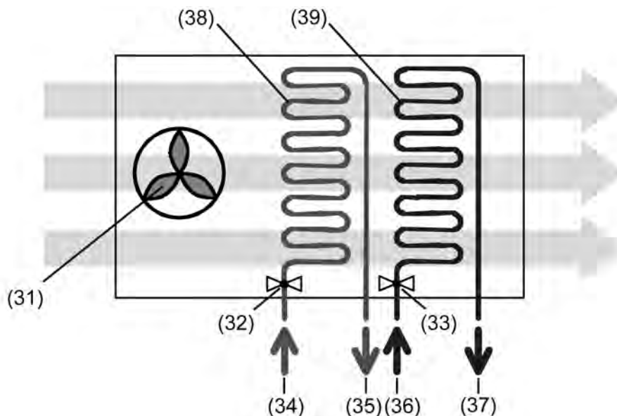
Bild 9: Das 4-Rohr-System
