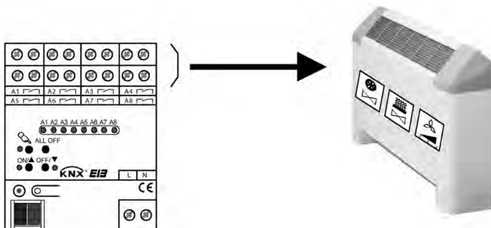
Bild 10: Der 1-Kanal-Betrieb
